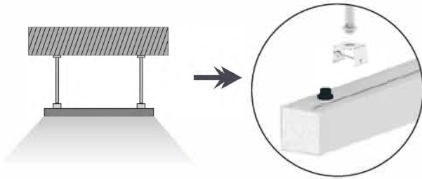
Pendant installation
